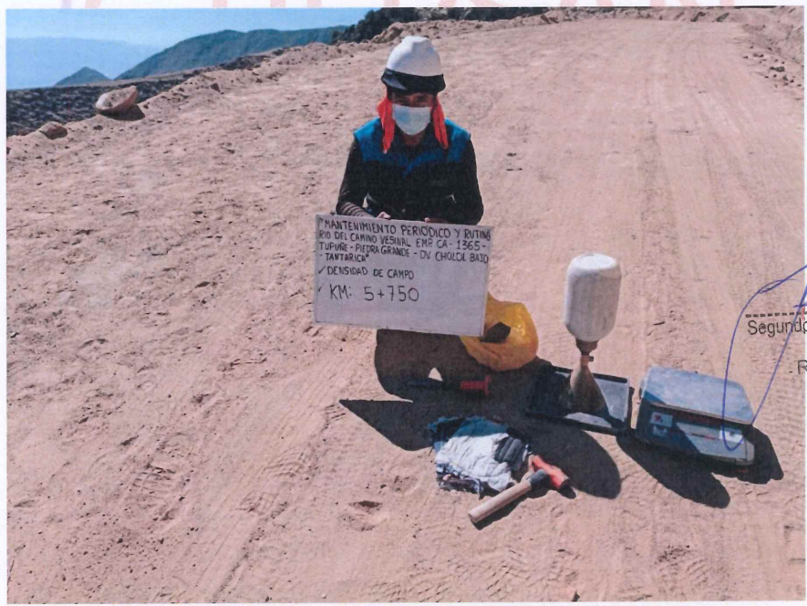
FIGURA N° 24. Ensayo de Densidad de Suelo en Campo. Progresiva 05 + 750 (Método del cono de arena).
