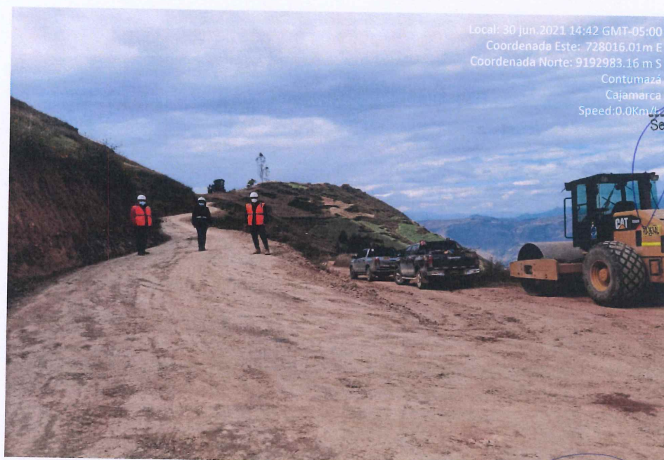
Fotografía 40. Resultado del refine y compactación del material granular para afirmado e=0.15m y verificación de los trabajos en campo por parte de la Entidad.
