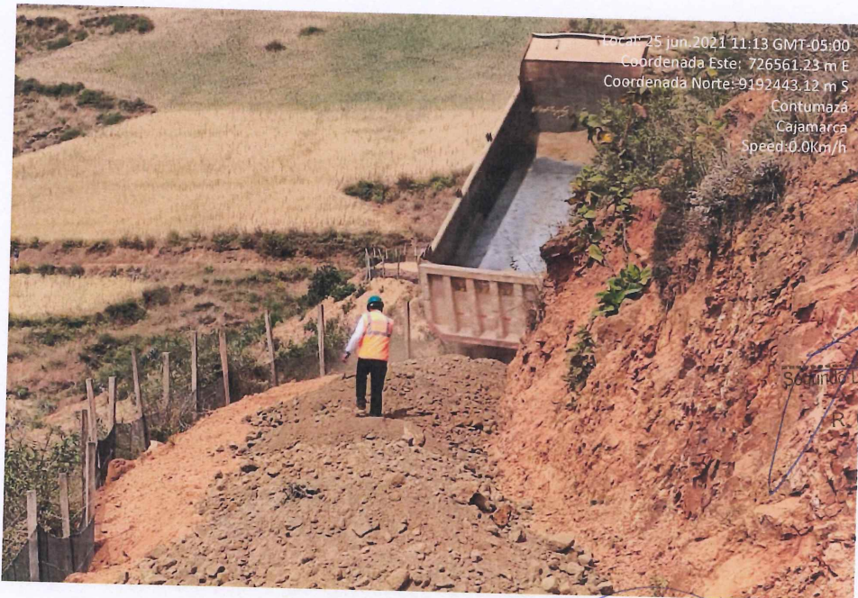
Fotografía 20. Descarga del material para el afirmado.
