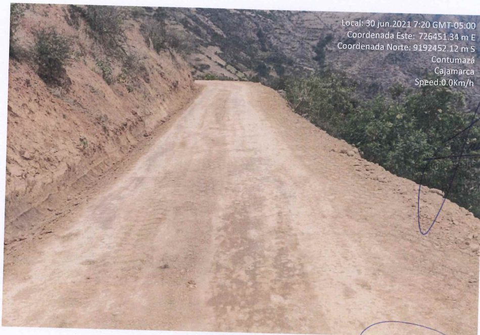
Fotografía 35. Resultado del refine y compactación de material granular para afirmado e=0.15m
