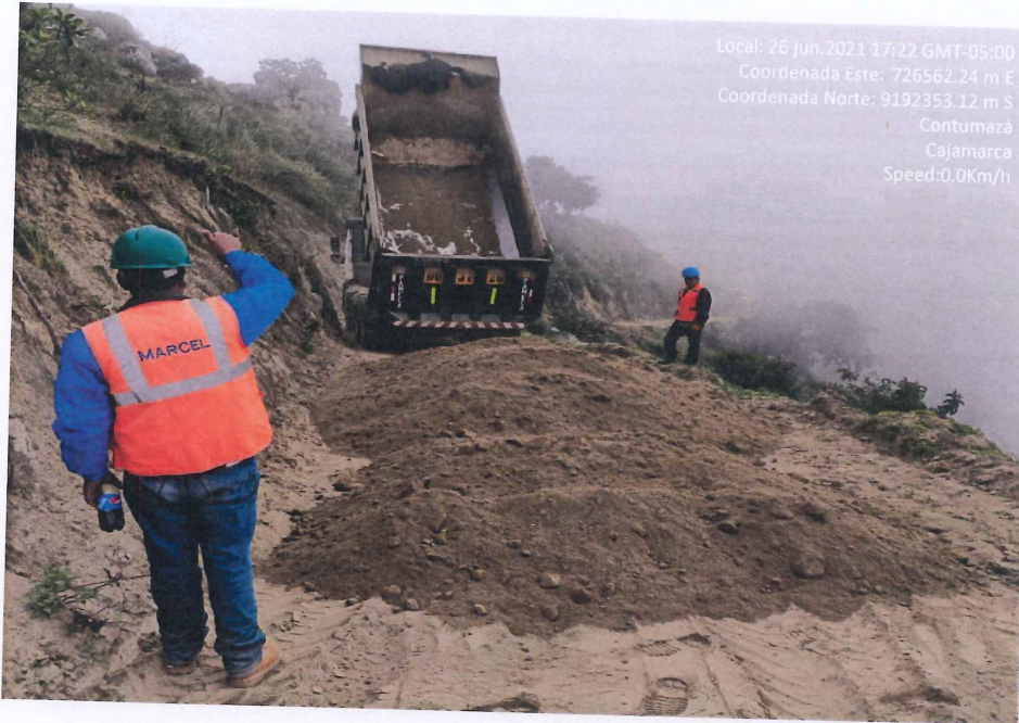
Fotografía 21. Descarga del material para el afirmado.
