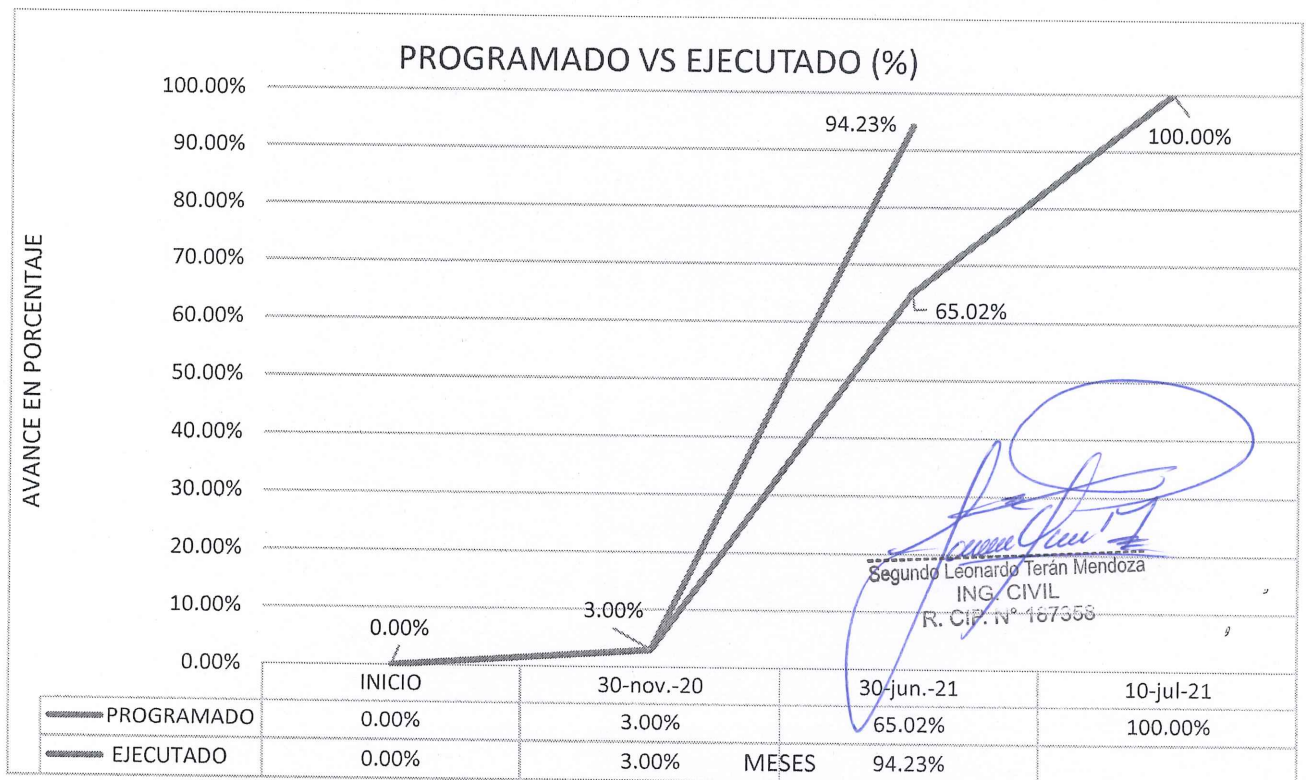
Gráfico de actividades programadas vs ejecutadas (Curva S)
