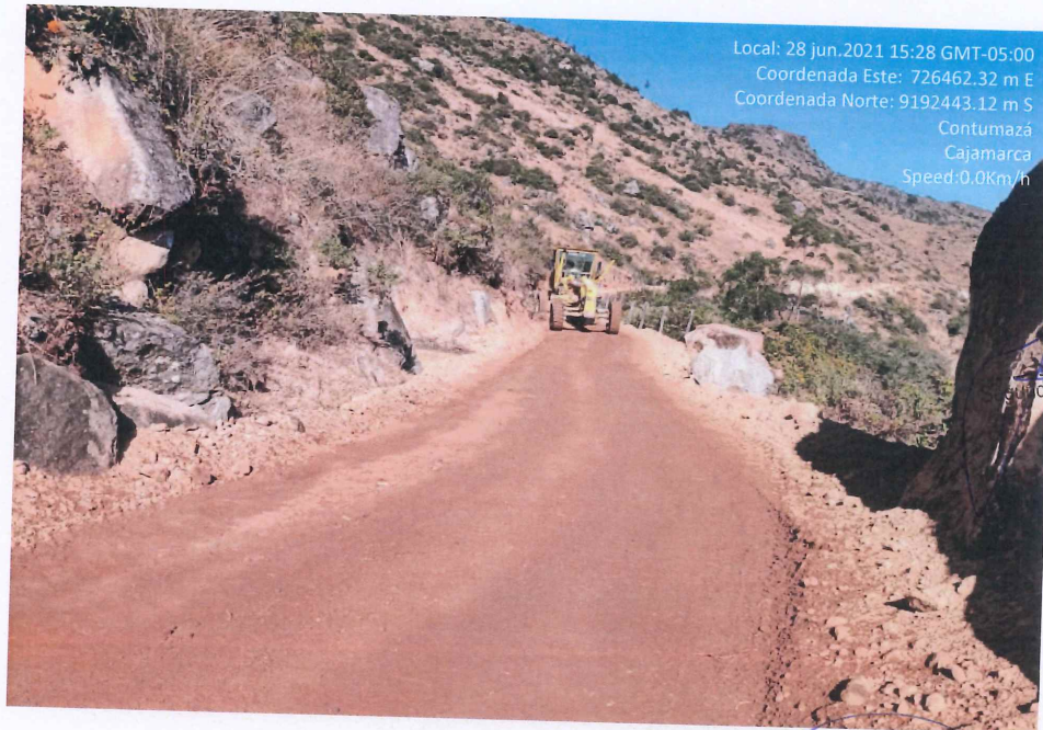
Fotografía 24. Conformación de la carpeta del afirmado y reconformación de cunetas.
