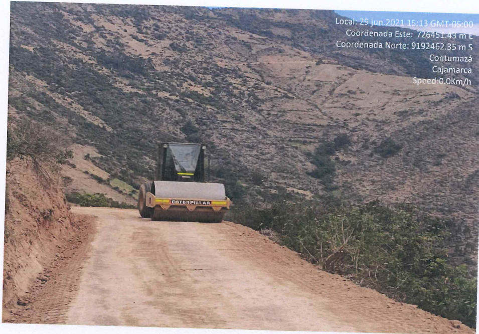
Fotografía 33. Refine y compactación de material granular para afirmado e=0.15m
