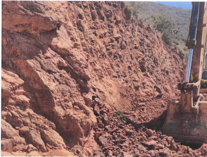
Fotografía N° 01: Vista general de la Cantera “TUPUÑE”.
