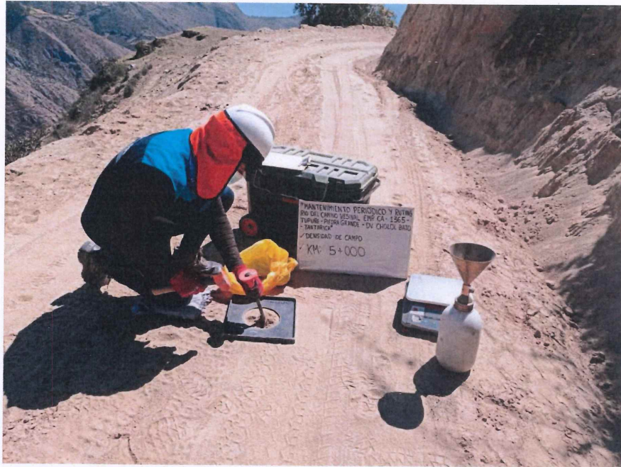
FIGURA N° 21. Ensayo de Densidad de Suelo en Campo. Progresiva 05 + 000 (Método del cono de arena).
