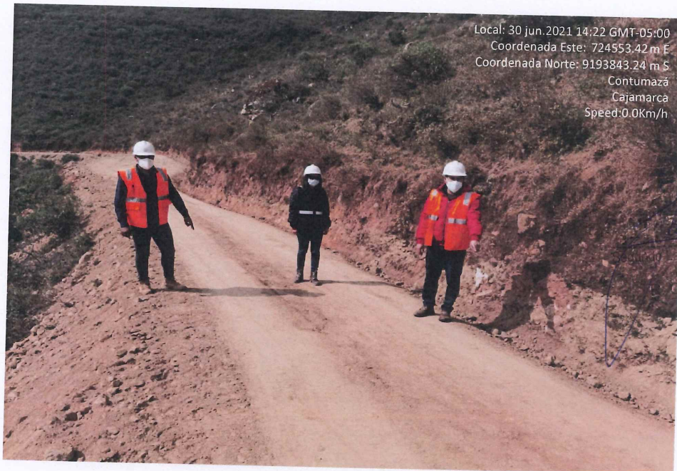
Fotografía 38. Resultado del refine y compactación del material granular para afirmado e=0.15m y verificación de los trabajos en campo por parte de la Entidad.
