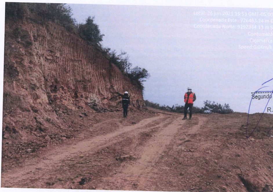
Fotografía 14. Resultado del ensanchamiento del camino vecinal con excavadora.
