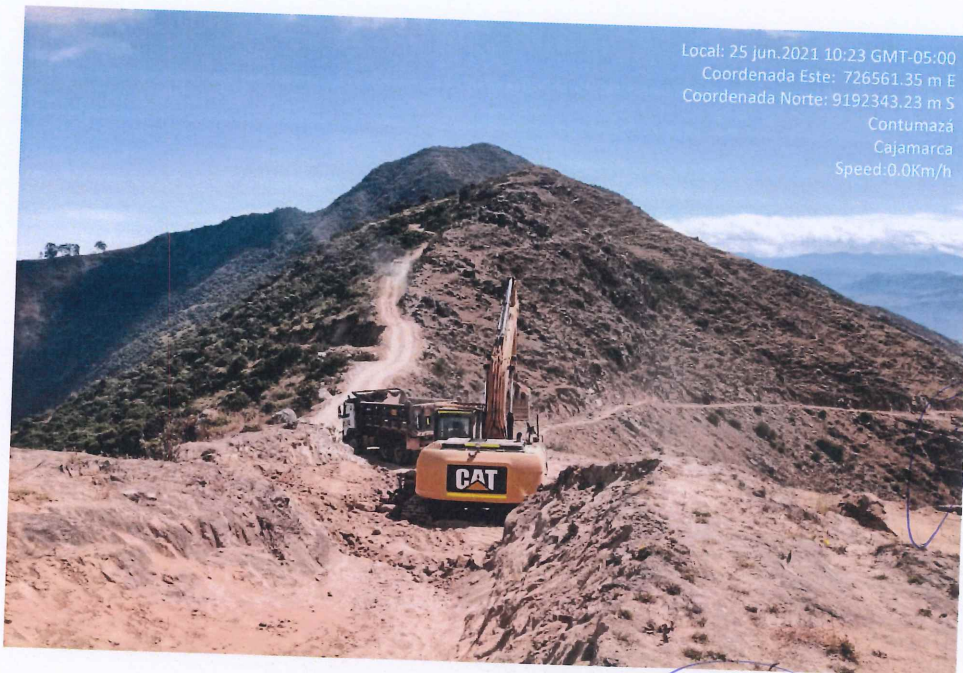
Fotografía 18. Carguío del material de cantera para el afirmado.
