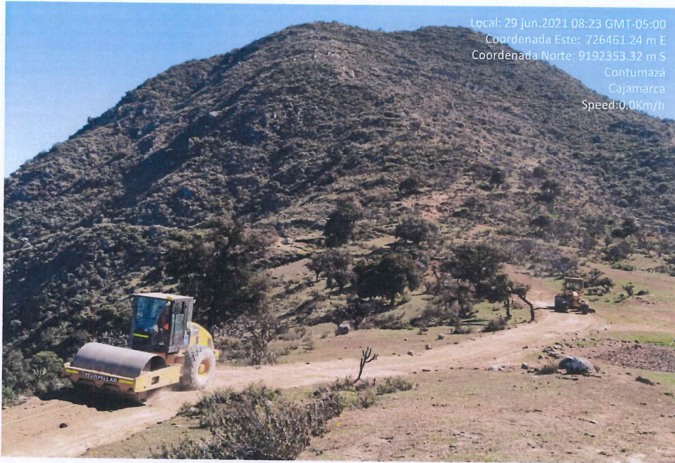
Fotografía 25. Conformación de la carpeta del afirmado y reconfirmación de cunetas.
